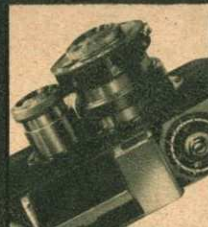
撮影レンズと反射ファインダーレンズとの聯動装置を示す
